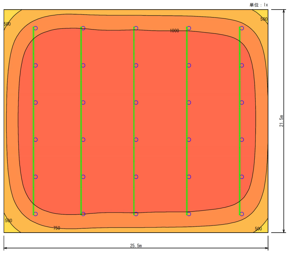
水平面照度分布図
