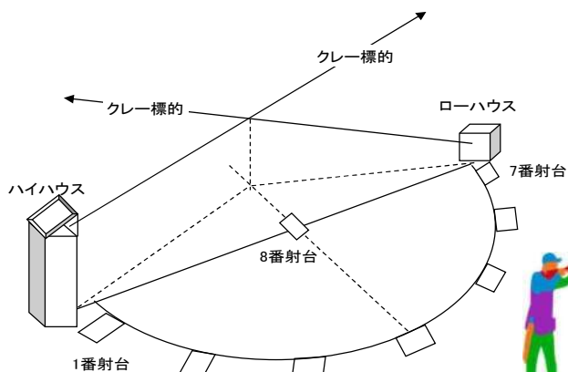
スキート射撃場立面構造図
