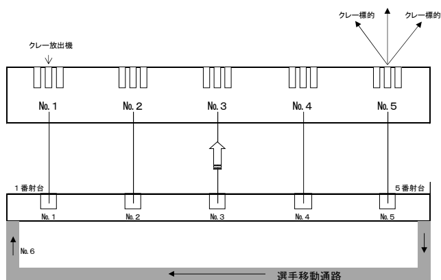
トラップ射撃場構造図
